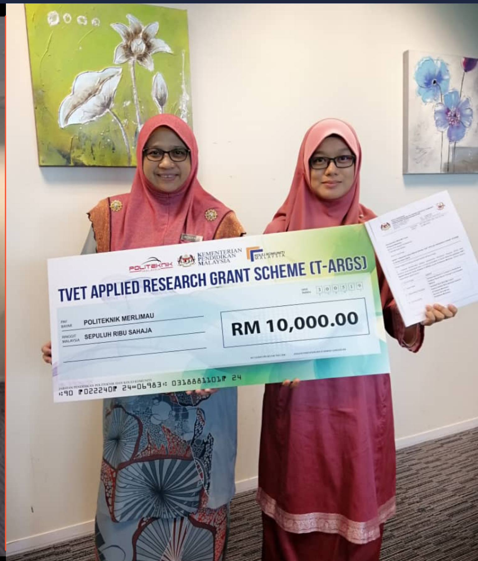
GERAN T-ARGS
